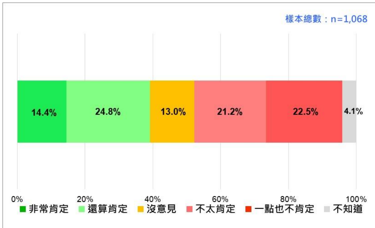
圖 2：國人對馬英九前總統大陸祭祖表現的感覺（2023/4）
