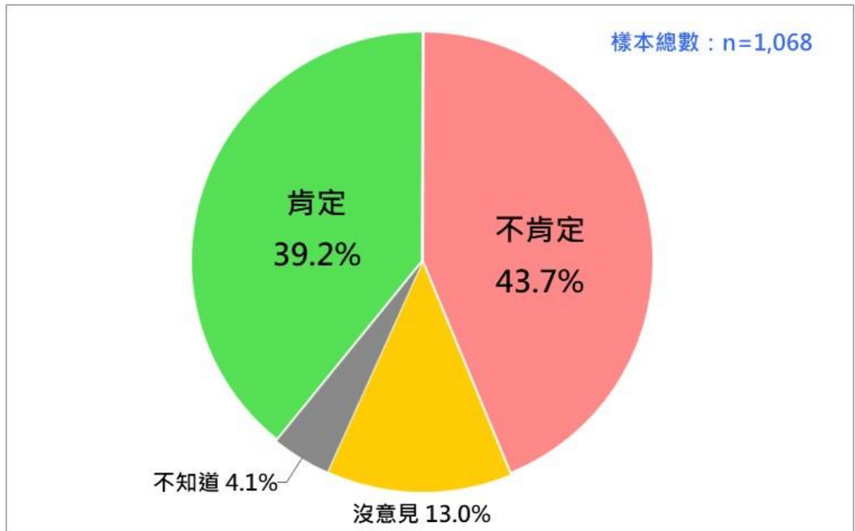
圖 1：國人對馬英九前總統大陸祭祖表現的感覺（2023/4）
